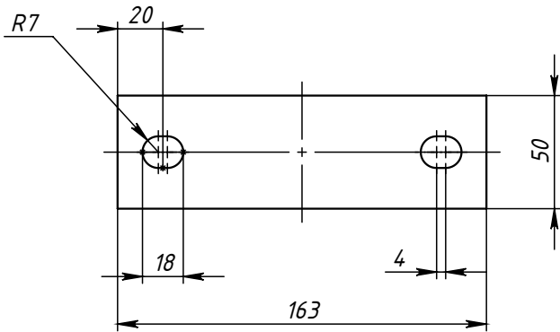
Поз.2 (Полухомут) развертка
